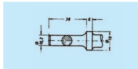
Vésőfej szárának mérete
