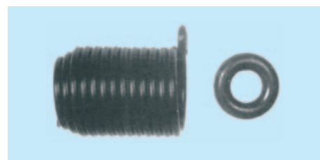
■ Biztonsági tartórugó és O-gyűrű UT 13/23 FHM ■ Bee hive spring and O-ring
