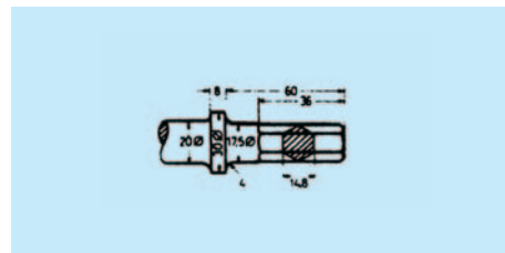
Vésőfej szárának mérete Dimensions Air Hammer
